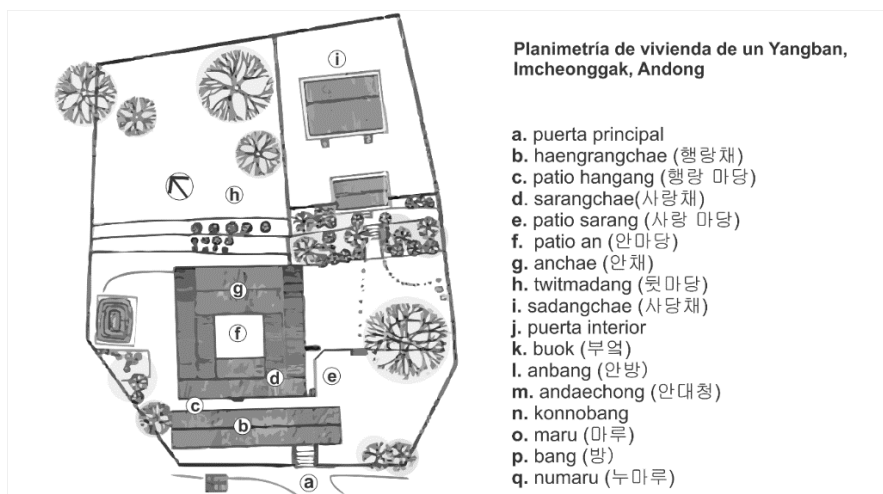
Imagen 2 Organization funcional de la vivienda
