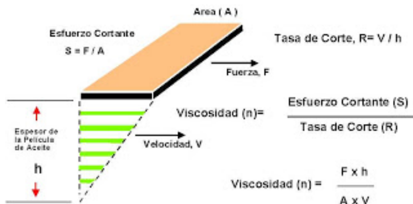
Figura 188: Viscosidad dinámica
