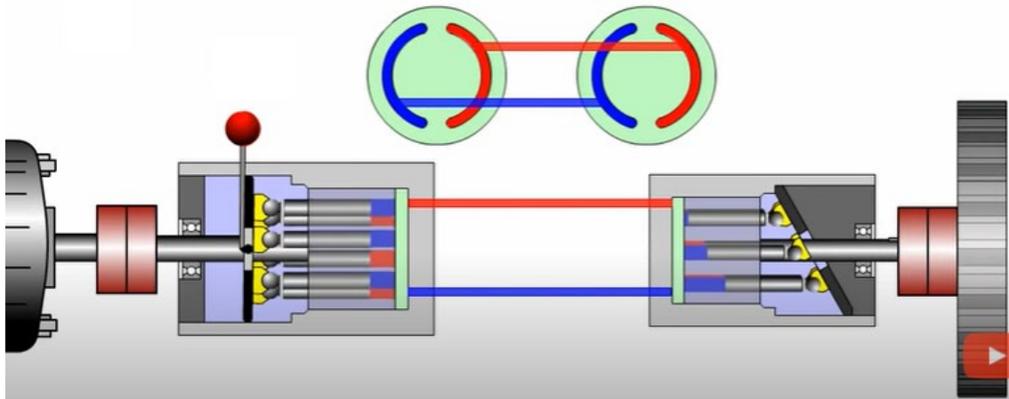
Figura 167: Transmisión hidrostática formada por una bomba de pistones (Izquierda) y un motor hidráulico (Derecha). En función de la posición de la placa de la bomba el eje conducido (vinculado al motor) va hacia adelante, hacia atrás o no se mueve
