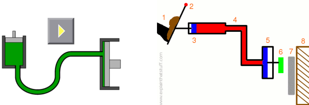
Figura 184: La presión hidráulica se puede transmitir por mangueras (Izquierda) Freno hidráulico (Derecha)
