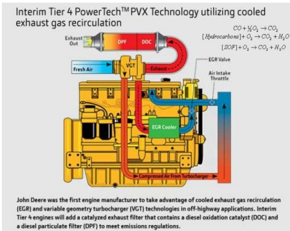
Figura 56: Esquema de motor John Deere con sistema de recirculación de gases de escape
