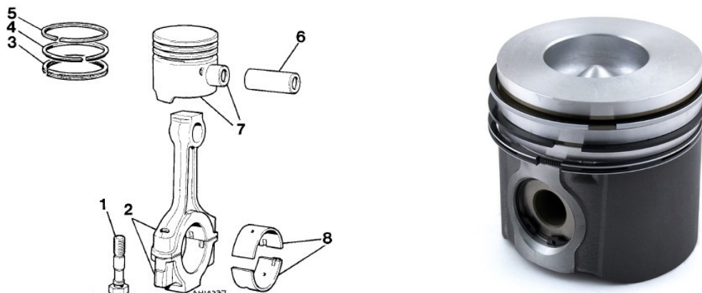
Figura 6: Izquierda: Pistón articulado en su parte inferior con la biela (2) a través del bulón (6) y en el que se aprecian los aros o segmentos (3, 4 y 5) y los cojinetes de biela (8) Derecha: Pistón típico de motor Diésel en el que se observa en la cabeza una excavación que corresponde a la cámara de combustión
