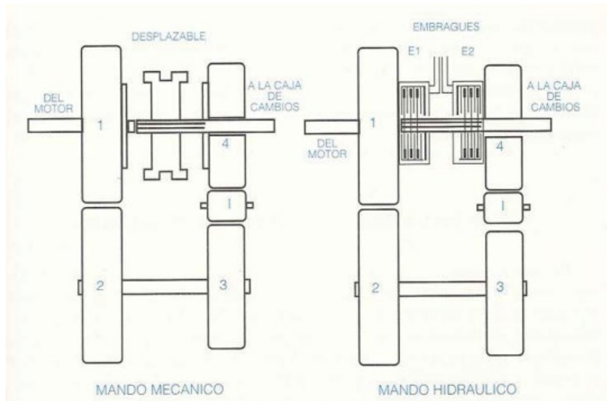
Figura 143: Inversor de sentido de avance de mando mecánico (Izquierda) e hidráulico (Derecha) (Adaptado de Arnal Atares y Laguna Blanca, 2000)
