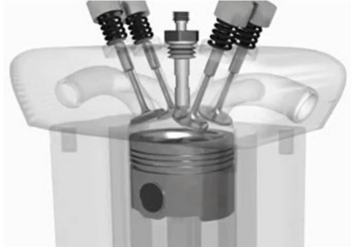
Figura 5: Ubicación de dos válvulas de admisión y dos de escape sobre la culata. En la parte central se encuentra el inyector
