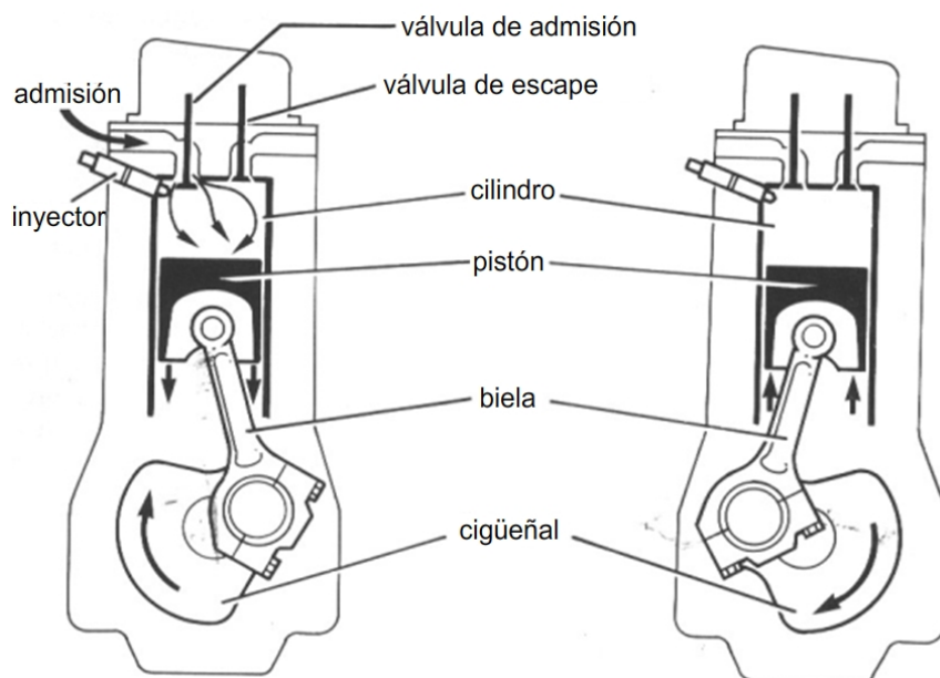
Figura 11: Tiempos del motor Diésel. Izquierda: Admisión (carrera descendente con la válvula de admisión abierta) Derecha: compresión (carrera ascendente con ambas válvulas cerradas)
