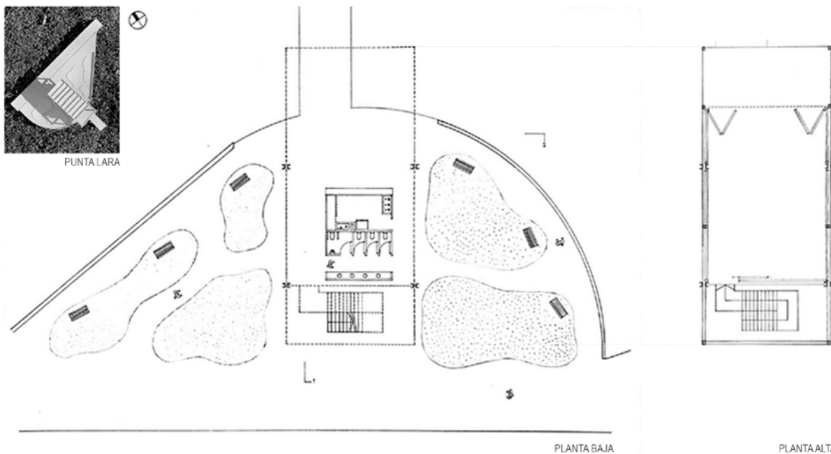
PLANTA BAJA
