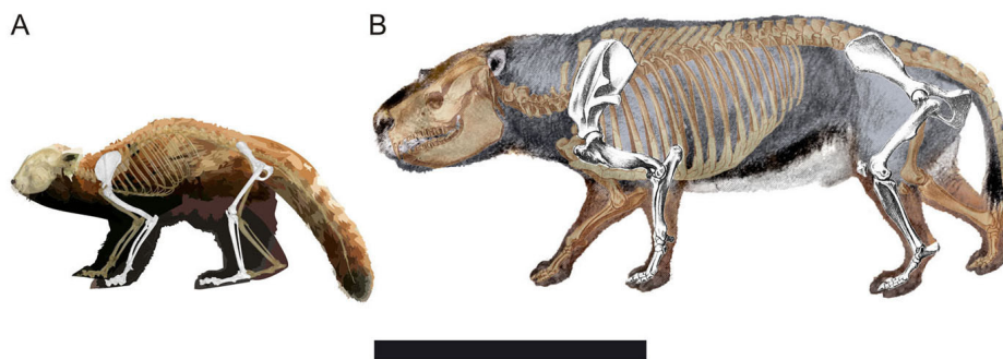
Figura III. 5. Vertebrados actuales y extintos con miembros no columnares. Los huesos del esqueleto apendicular, resaltados en blanco, se disponen en ángulo. A, panda rojo ( Ailurus ); B, notoungulado del Mioceno, Adinotherium (modificada de la ilustración de Robert Bruce Horsfall publicada en Scott, 1913). Escala= 50 cm
