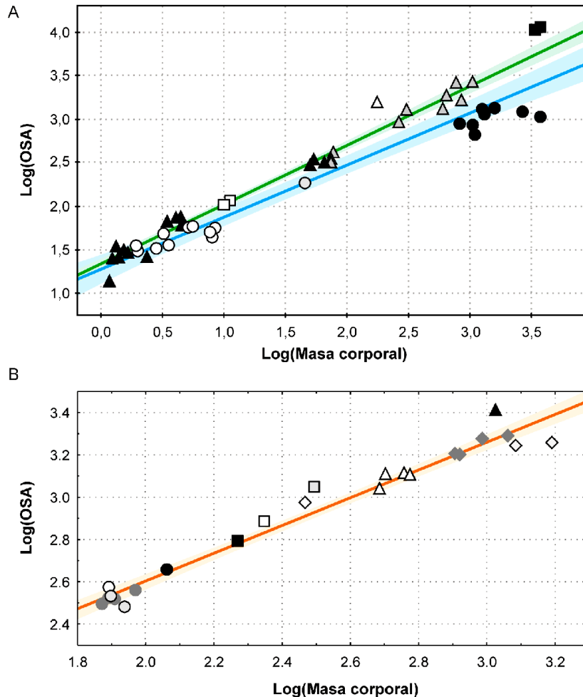
Figura VIII.25. Relación entre el área de la superficie ocular dentaria y la masa corporal en xenar-tros. A, xenar-tros actuales y extintos. Línea verde, regresión para los Cingulata; línea azul regresión para los Folivora. Símbolos: triángulos negros, cingulados dasipódidos; triángulos grises, cingu-lados pampatéridos; triángulos blancos, cingula-dos gliptodóntidos; círculos blancos, tardígrados actuales; círculos grises, Eucholoeops (tardígrado Mioceno); cuadrados blancos, Hapalops (tardígrado Mioceno); cuadrados negros, Megatherium ; círculos negros, milodóntidos. Modificado de Vizcaino et al. (2006). B. Gliptodontes. Línea roja, regresión. Símbolos: círculos blancos, Asterostemma (Mio-ceno); círculos grises con borde negro Cochlops (Mioceno); círculos negros Eucinepeltus (Mioceno); círculos gris oscuro, Propalaeohoplophorus (Mioceno); cuadrado blanco, Hoplophractus (Mio-Plioceno); cuadrado gris Neuryurus (Plioceno temprano), cuadrado negro, Eosclerocalyptus (Mio-Plioceno), triángulos blancos, Neosclerocalyptus (Pleistoceno); triángulo negro, Panochthus (Pleistoceno); rombo blanco, Urotherium (Pleistoceno), rombos grises con borde negro, Doedicurus (Pleistoceno); rombos gris oscuro, Glyptodon (Pleistoceno). Modificado de Vizcaino et al. (2011). Áreas som-breadas alrededor de las líneas de regresión = in-tervalo de confianza del 95%.
