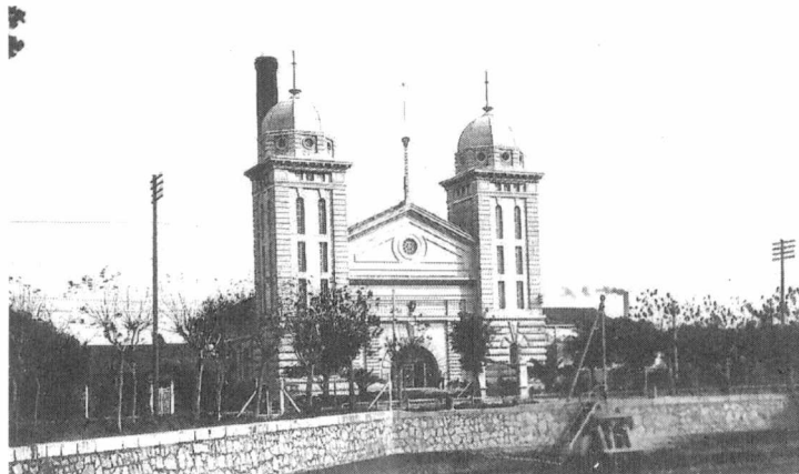
Antigua Usina Hidráulica, frente al dock central del Puerto La Plata, desde donde se movían por presión hidráulica los guinches y cabrestantes del puerto. De magnífica dimensión y expresión arquitectónica. Fotografía: propiedad de Gladys Guiamet.
